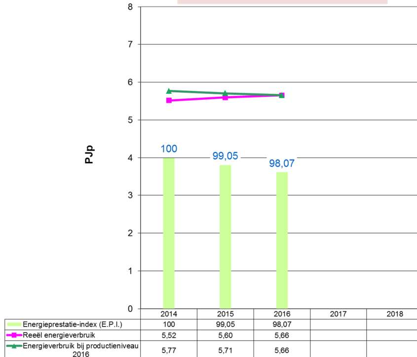
Grafiek 44: Evolutie 2014 – 2016 van het energieverbruik en de E.P.I. voor Textiel & Hout (niet VER-bedrijven)
