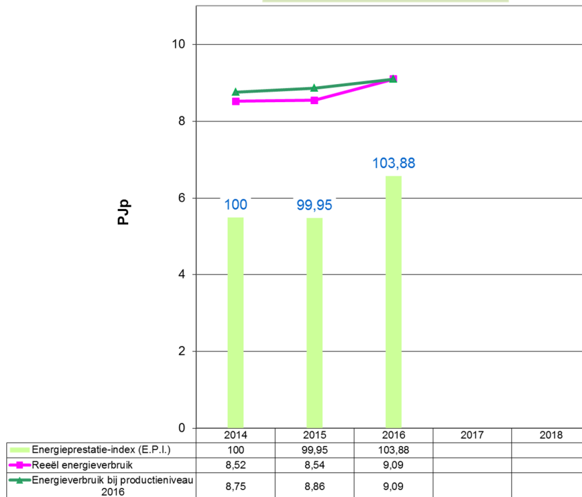
Grafiek 43: Evolutie 2014 – 2016 van het energieverbruik en de E.P.I. voor Textiel & Hout (VER-bedrijven)
